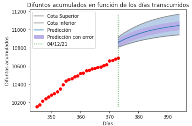
Figura 6. En los puntos rojos se muestran el número de difuntos acumulados reportados desde el 11 de marzo del 2021 hasta el 12 de abril del 2021. En la región azul se encuentran los valores predichos para los siguientes veintidós días.
