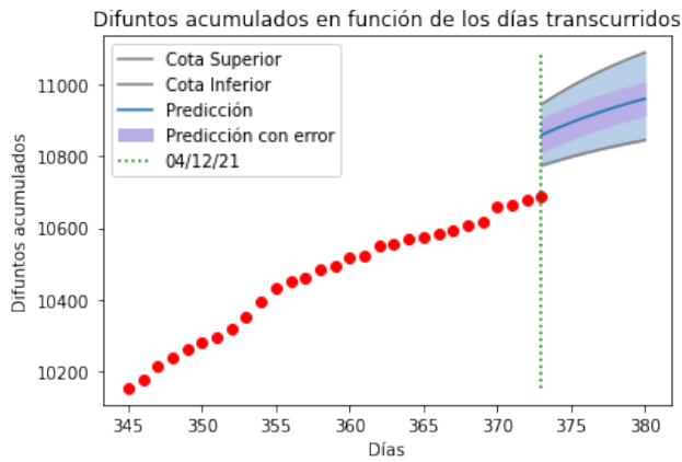
Figura 3. En los puntos rojos se muestran el número de difuntos acumulados reportados desde el 11 de marzo del 2021 hasta el 12 de abril del 2021. En la región azul se encuentran los valores predichos para los siguientes siete días.
