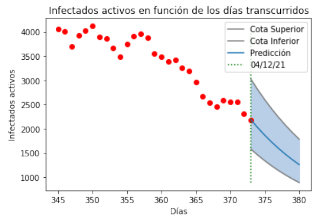
Figura 1. En los puntos rojos se muestran los casos infectados activos calculados, día a día, desde el 11 de marzo del 2021 hasta el 12 de abril del 2021. En la región azul se encuentran los valores predichos en los siguientes siete días.
