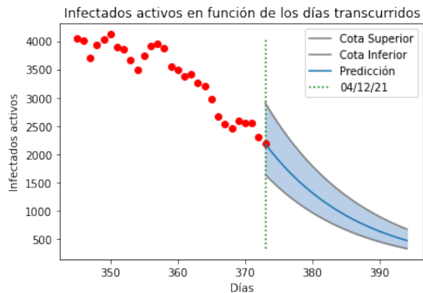
Figura 4. En los puntos rojos se muestran los casos infectados activos calculados, día a día, desde el 11 de marzo del 2021 hasta el 12 de abril del 2021. En la región azul se encuentran los valores predichos para los siguientes veintidós días.
