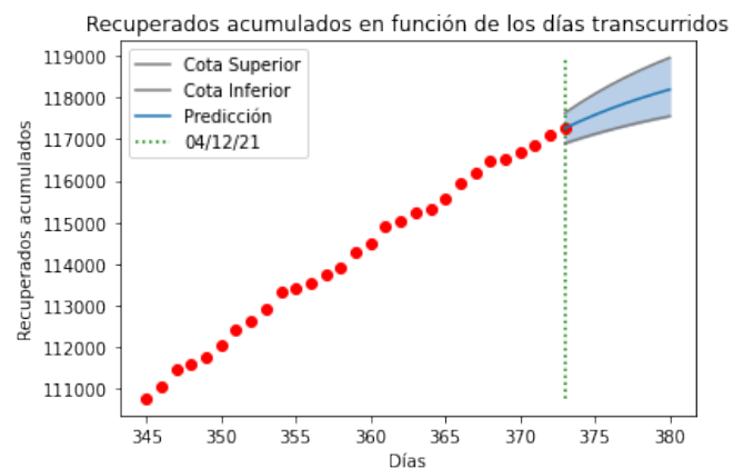
Figura 2. En los puntos rojos se muestran los casos recuperados acumulados reportados desde el 11 de marzo del 2021 hasta el 12 de abril del 2021. En la región azul se encuentran los valores predichos para los siguientes siete días.
