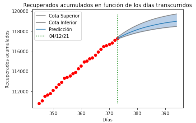
Figura 5. En los puntos rojos se muestran los casos recuperados acumulados reportados desde el 11 de marzo del 2021 hasta el 12 de abril del 2021. En la región azul se encuentran los valores predichos para los siguientes veintidós días.
